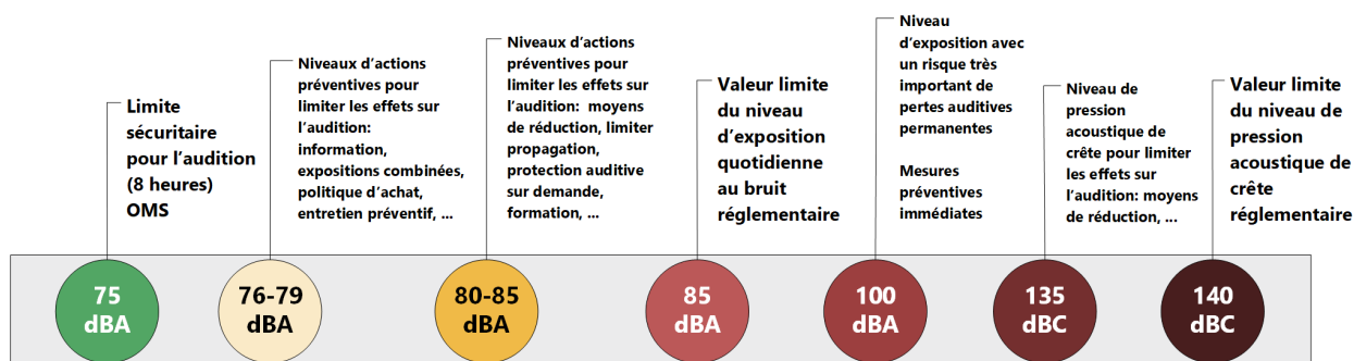
Figure 6 Résumé des niveaux d'actions préventives et des valeurs limites d'exposition réglementaires au bruit en milieu de travail
