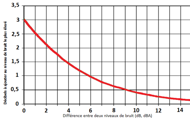
Figure A-9 Abaque pour l'addition de deux niveaux de bruit
